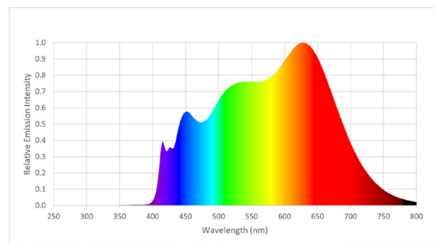
CRI 95 - 4000 K
