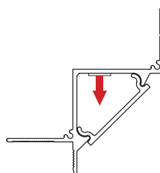
Iluminación directa
