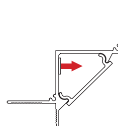
Iluminación indirecta
